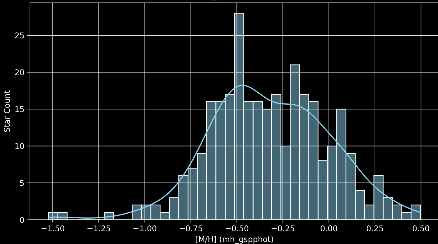
GALAH DR4 Field: [6960] [M/H] (mh_gspphot) (n= 302)
