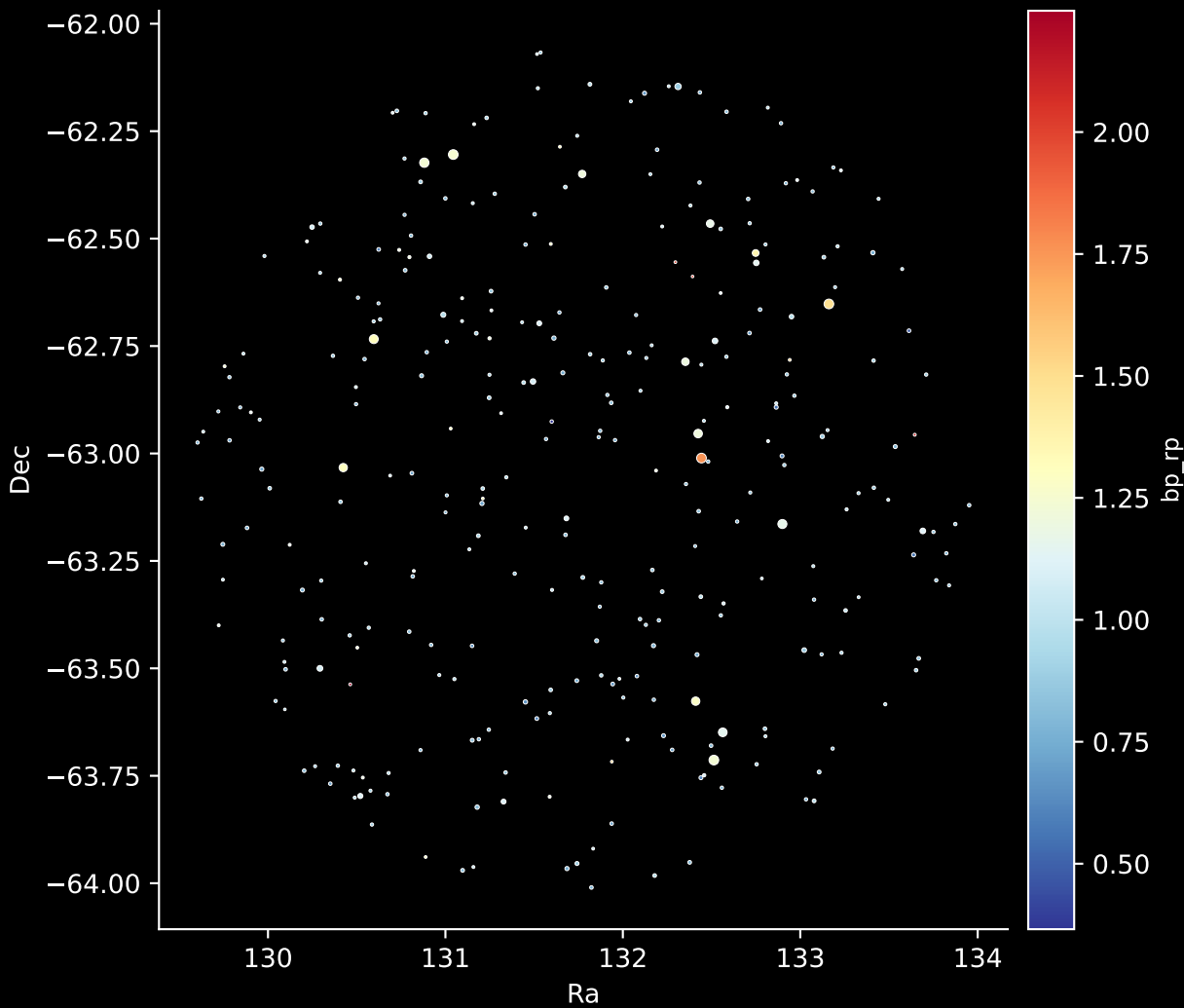
GALAH DR4 Field: [6960] Stars: 302
