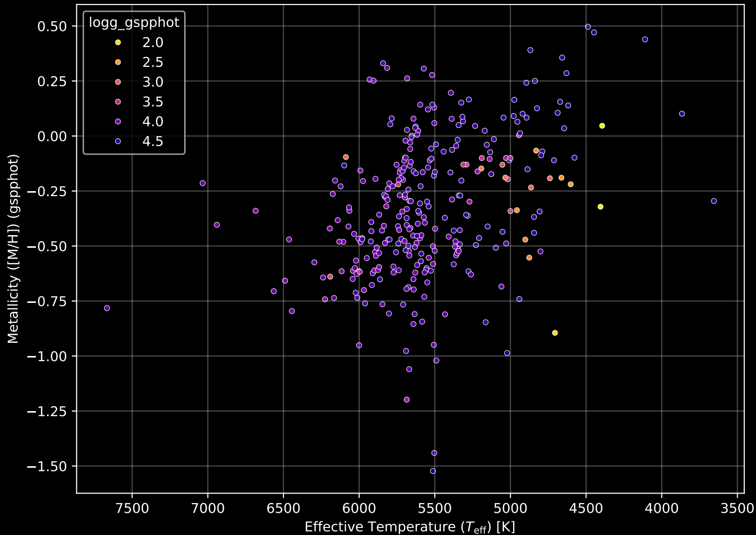
GALAH DR4 Field: [6960] Stellar Population Parameters (n= 302)
