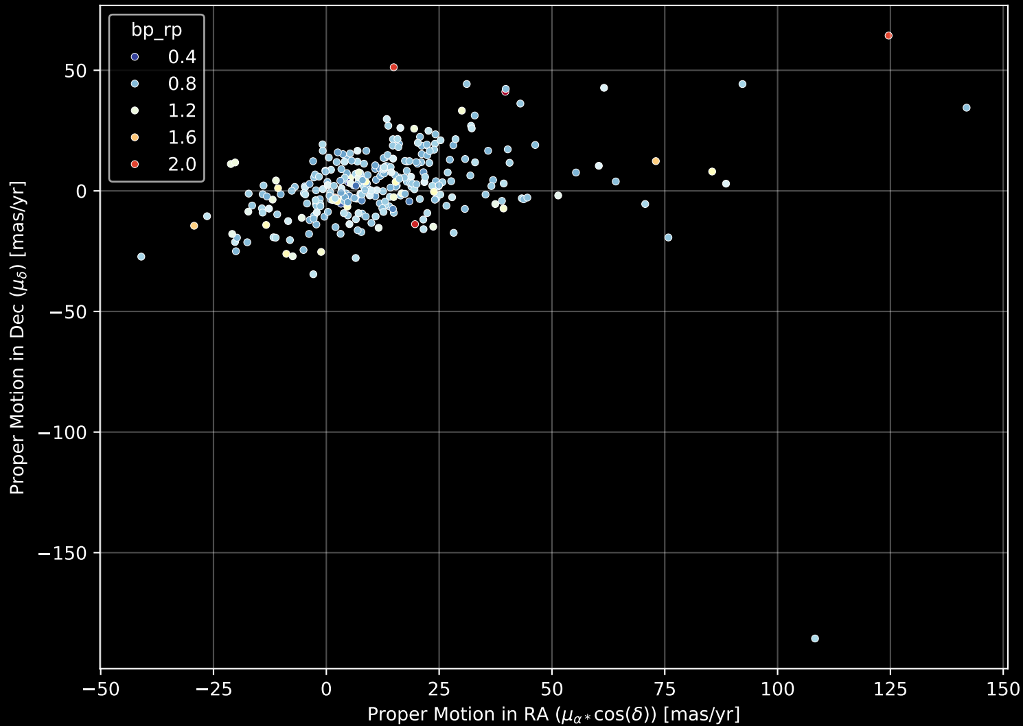
GALAH DR4 Field: [6960] Proper Motion Diagram (n= 302)
