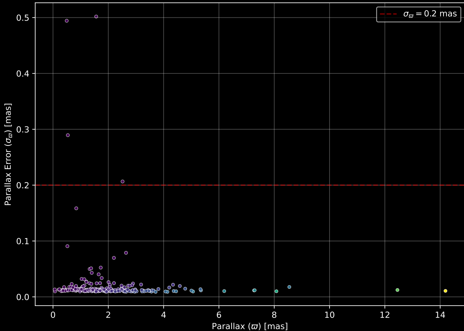
GALAH DR4 Field: [6960] Parallax Quality (n= 302)
